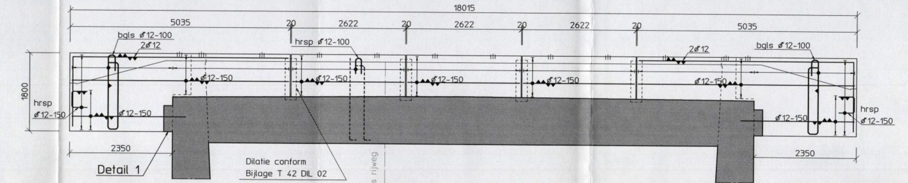
Doorsnede F
