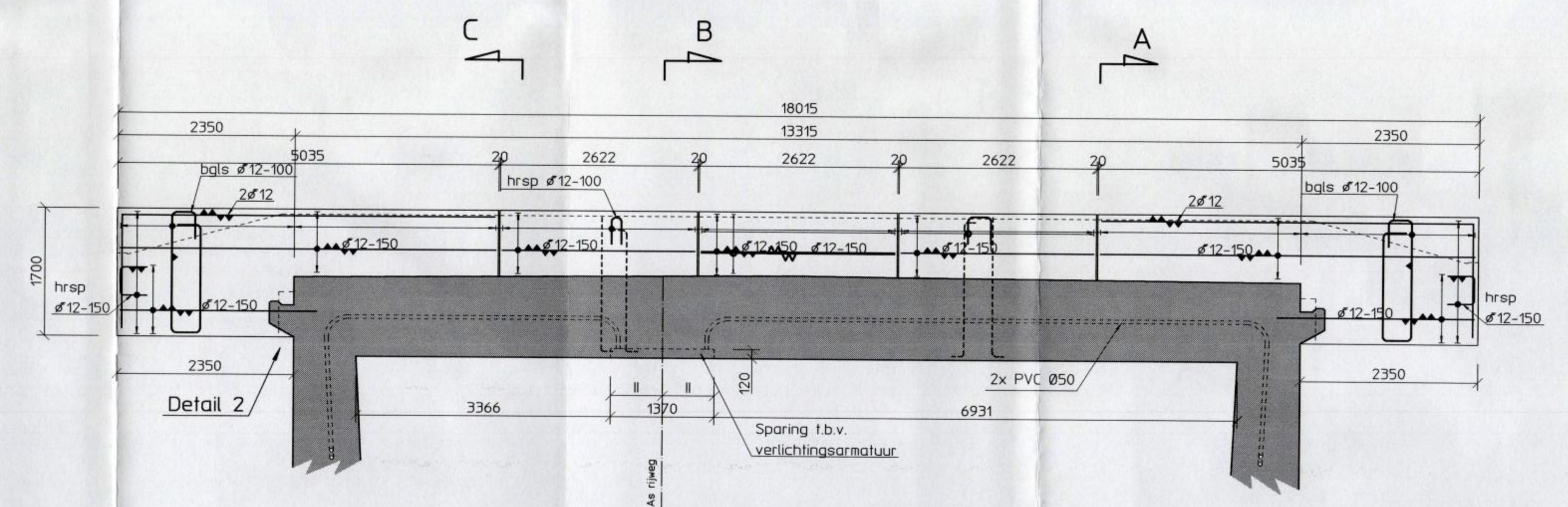
Doorsnede G
