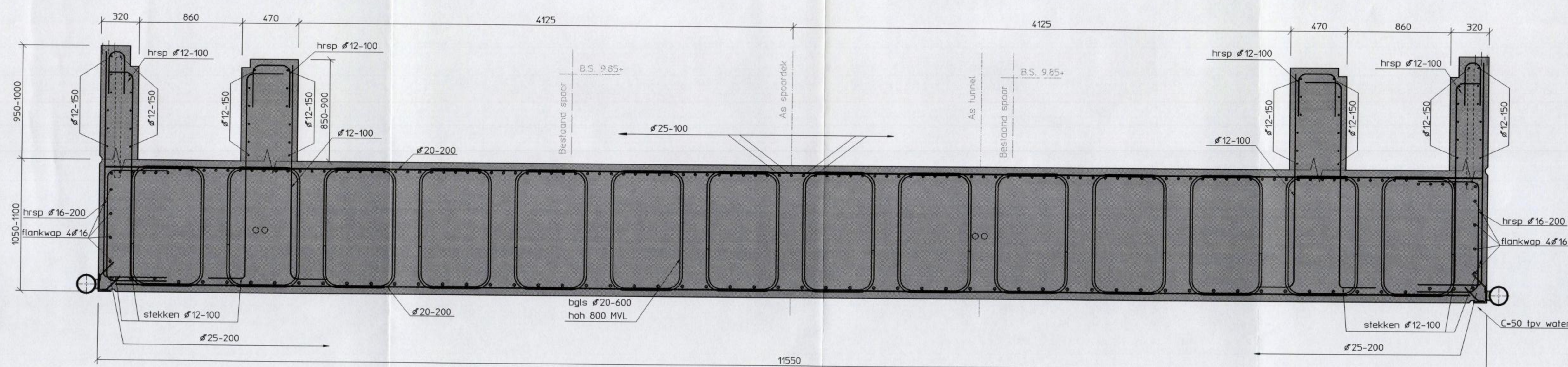
Doorsnede I
