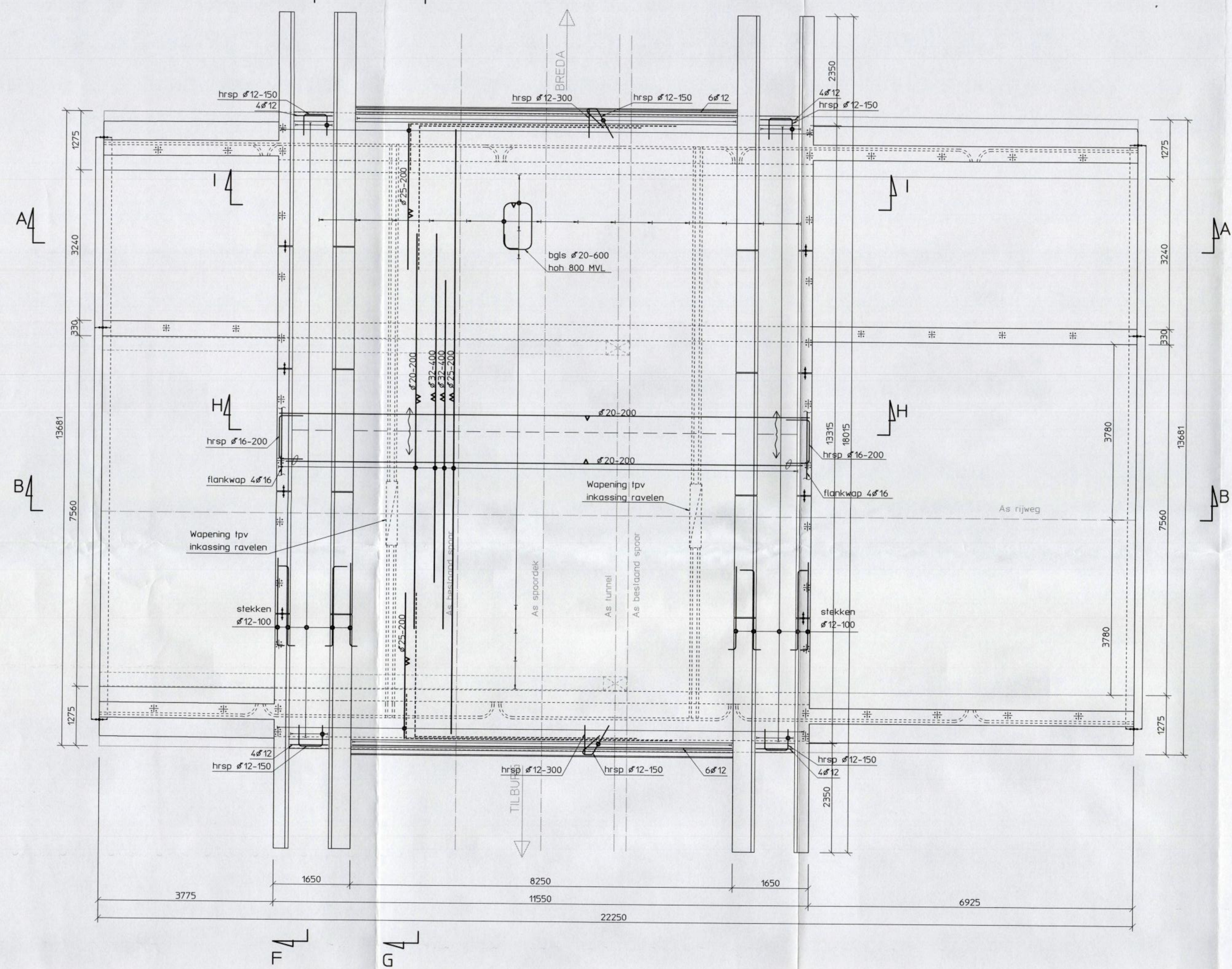
Bovenaanzicht
